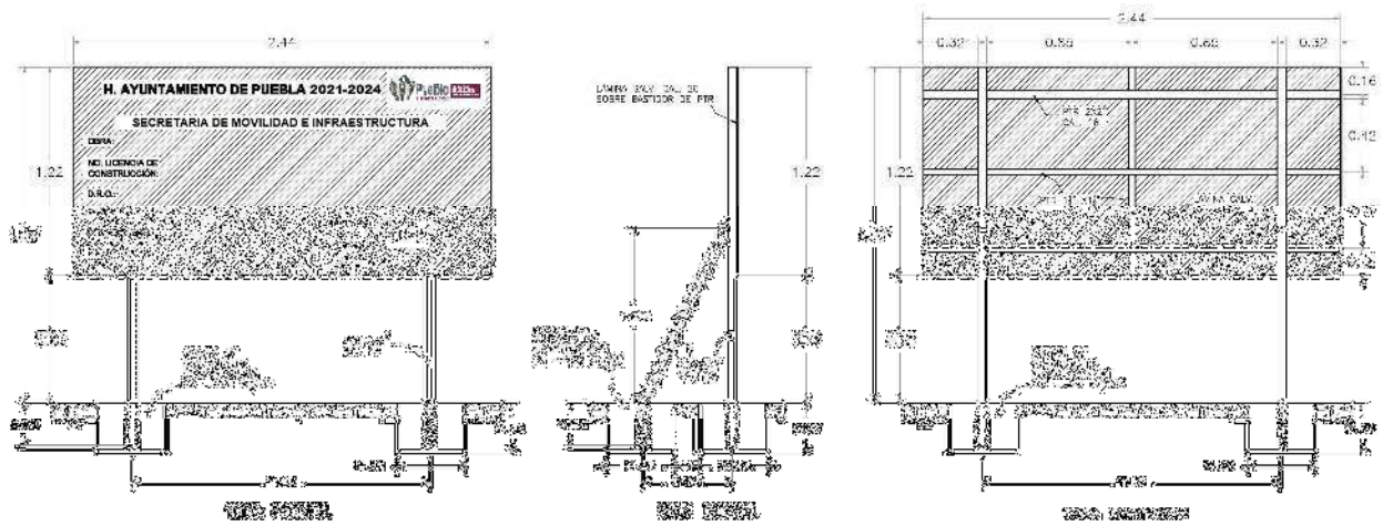
DETALLE DE LA LONA INFORMATIVA PARA LA OBRA DE LA DEPENDENCIA CONTRATANTE
