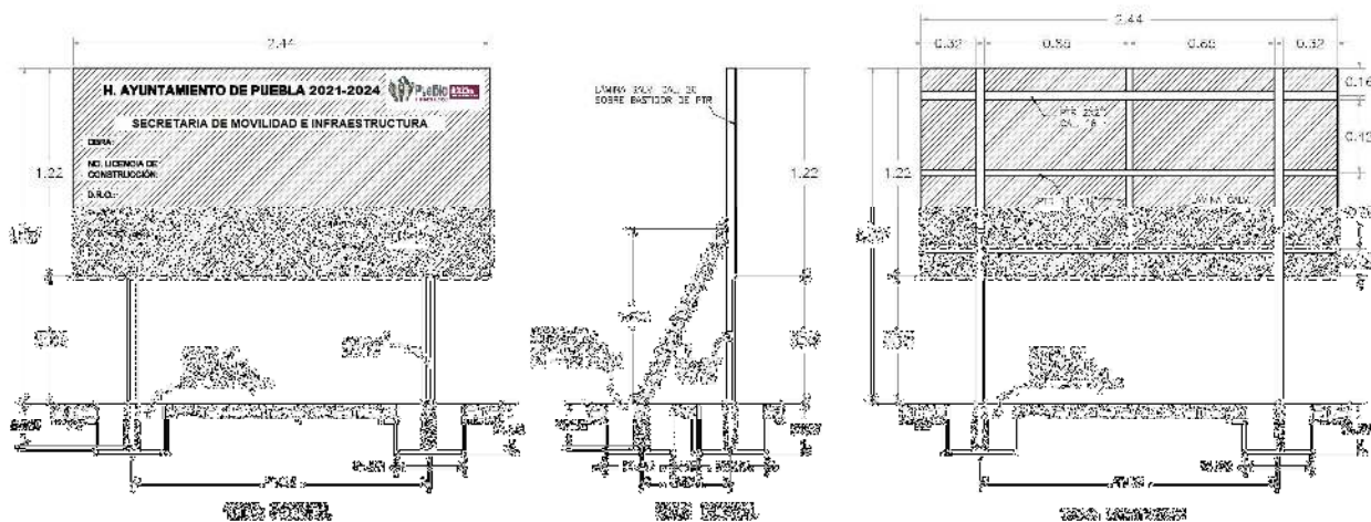
LETRERO INFORMATIVO DE LA OBRA (VISTA LATERAL)
