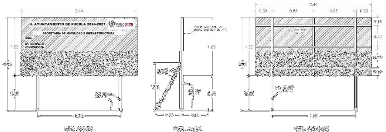
LETRERO INFORMATIVO DE LA OBRA (VISTA FRONTAL)
